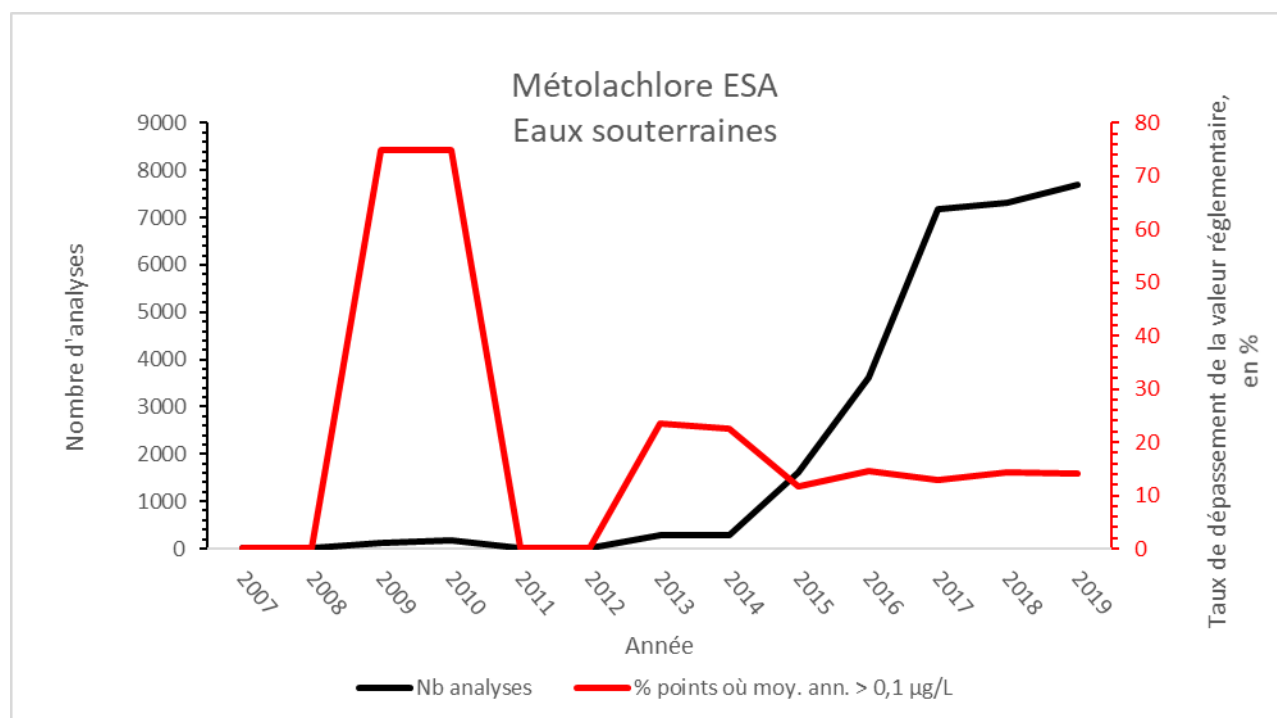
Figure 19 : Nombre d'analyses et taux de dépassement de la valeur réglementaire (0,1 µg/L) du métolachlore ESA (CGA 354743), dans les ESO de métropole, sur la période 2007-2019.
