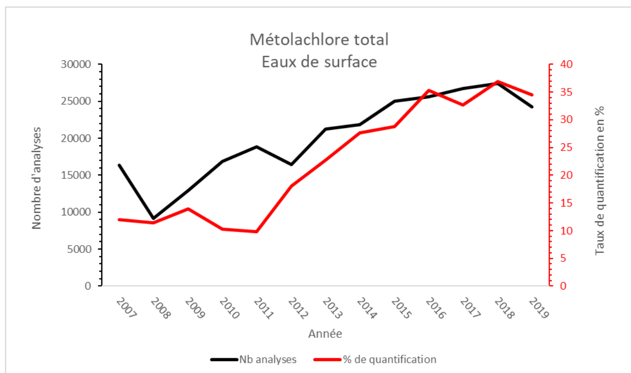
Figure 5 : Nombre d'analyses et taux de quantification du métolachlore total, dans les ESU de métropole, sur la période 2007-2019.
