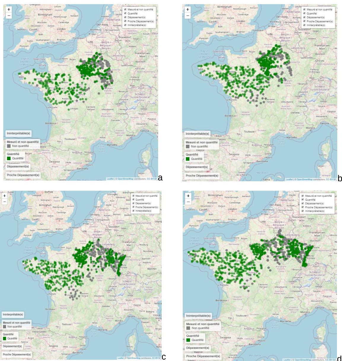
Figure 15 : Répartition des points de surveillance des eaux de surface pour lesquelles le métolachlore NOA 413173 (SYN 547627) a été mesuré au moins 4 fois par an (gris), quantifié au moins une fois (vert), pour les années 2016 (a), 2017 (b), 2018 (c) et 2019 (d).
